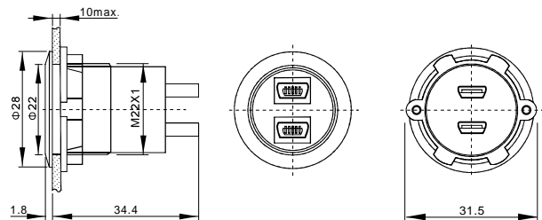
产品描述 : Mini USB2.0 2×B型母/B型公 Product Description: Mini USB2.0 2×FEMALE B/ MALE B
