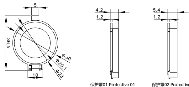
保护罩01 Protective 01
