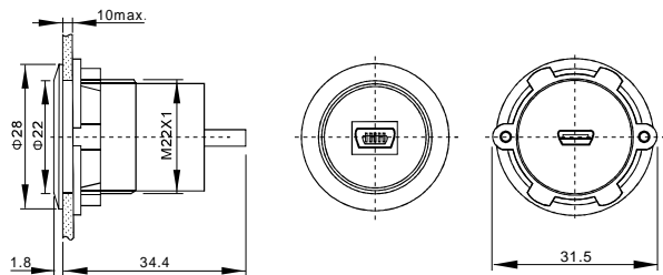
产品描述 : Mini USB2.0 B型母/B型公 Product Description: Mini USB2.0 FEMALE B/ MALE B
